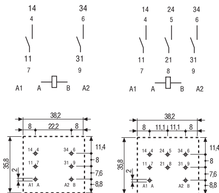
62.22 - 4300 62.23 - 4300 pohled ze strany vývodů pohled ze strany vývodů
