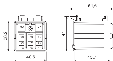
062.08 s relé 62.3x.x.xxx.xxx0 nebo 62.8x.x.xxx.xxx9
