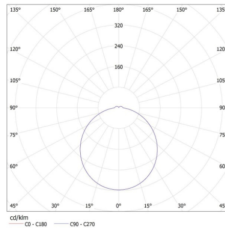
KANLUX S.A. (kat 26440) VARSO LED 18W-WW-O / Krzywa rozsytu światła (biegunowo)
