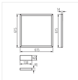
AVAR 6262 40W
