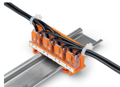
Odlehčení tahu pomocí vázacích pásek na upevňovacím adaptéru (příčně vůči směru zapojení vodičů) – kontaktní místa označená popisovacími pásky (210-334)
