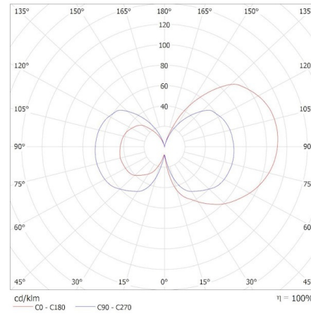
KANLUX S.A. (kat 29605) XLED A60 10W-WW / Krzywa rozsytu światła (biegunowo)
