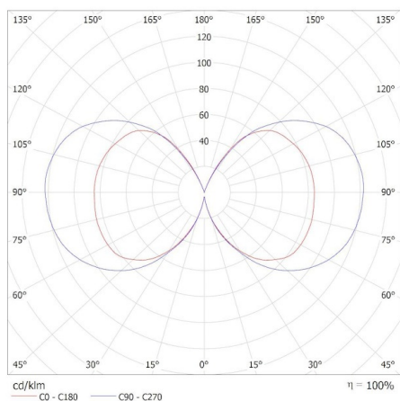
KANLUX S.A. (kat 39600) XLED A60 4,5W-WW / Krzywa rozsyłu światła (biegunowo)
