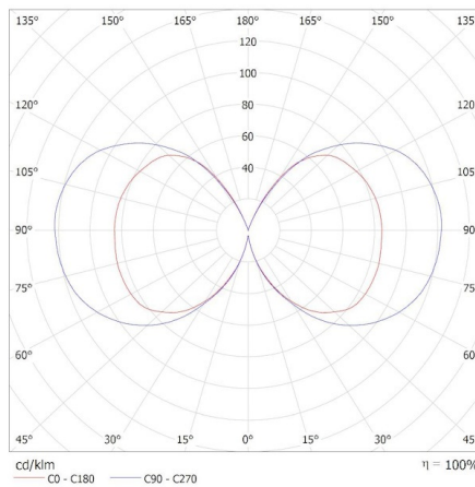
KANLUX S.A. (kat 39600) XLED A60 4,5W-WW / Krzywa rozsytu światła (biegunowo)
