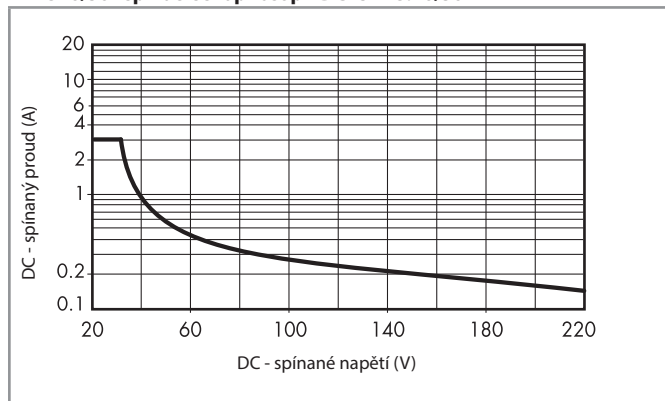
H 7S16/36 - spínací schopnost při DC13 - 7S.16/36
