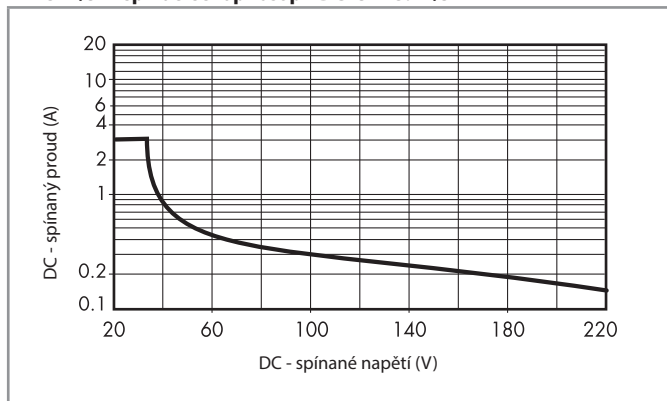
H 7S14/34 - spínací schopnost při DC13 - 7S.14/34
