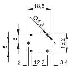
pohled ze strany vývodů
