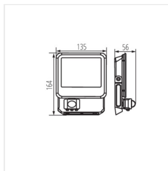
IQ-LED FL-10W-NW-SE
