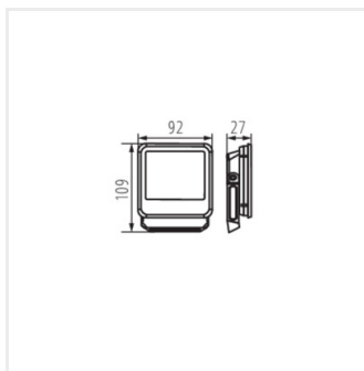
IQ-LED FL-10W-NW
