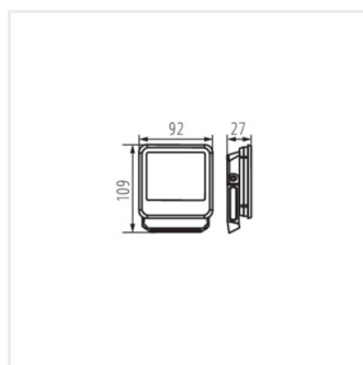
IQ-LED FL-10W-NW
