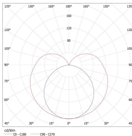
KANLUX S.A. (kat 26360) ALDO 4LED 1X60 + Miledo / Krzywa rozsyłu światła (biegunowo)
