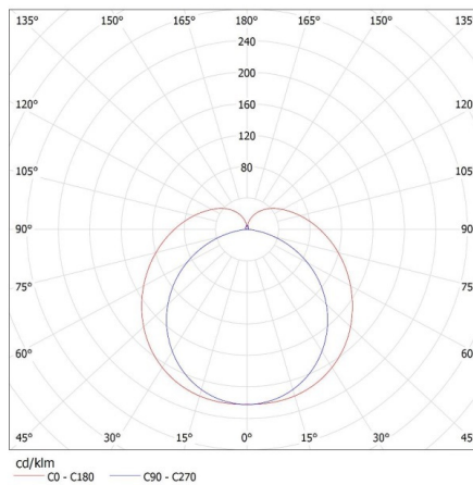
KANLUX S.A. (kat 26700) ROLSO LED IP44 15W-NW / Krzywa rozsytu światła (biegunowo)
