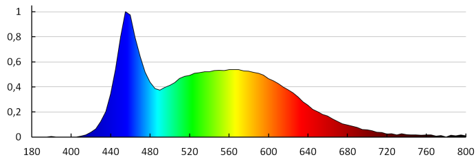
KANLUX S.A. (kat 23110) SABI LED CW / LDC (Polar)
