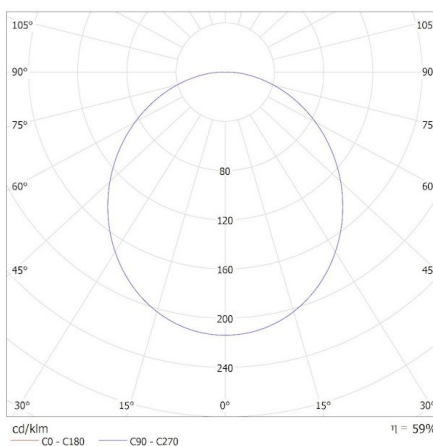
KANLUX S.A. (kat 38383) BENO ECO 20W CCT O B 3000K / Krzywa rozsyłu światła (biegunowo)
