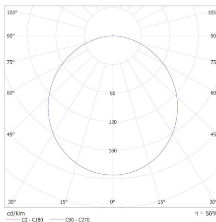
KANLUX S.A. (kat 38385) BENO ECO 30W CCT O B 3000K / Krzywa rozsyłu światła (biegunowo)
