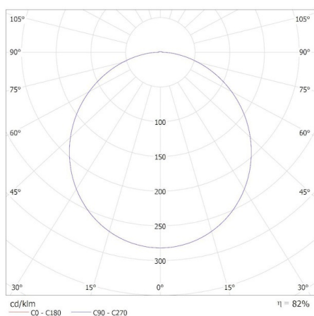
KANLUX S.A. (kat 38384) BENO ECO 30W CCT O W 4000K / Krzywa rozsyłu światła (biegunowo)
