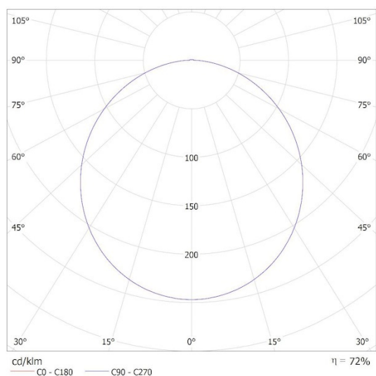
KANLUX S.A. (kat 38386) BENO ECO 40W CCT O W 3000K / Krzywa rozsyłu światła (biegunowo)
