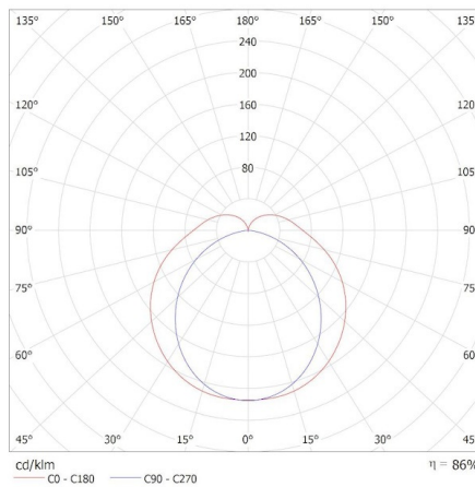
KANLUX S.A. (kat 36661) AKVO IP44 15W-NW-C / Krzywa rozsytu światła (biegunowo)
