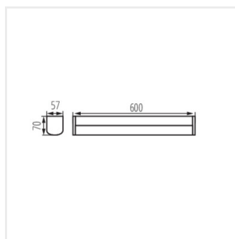
AKVO IP44 15W
