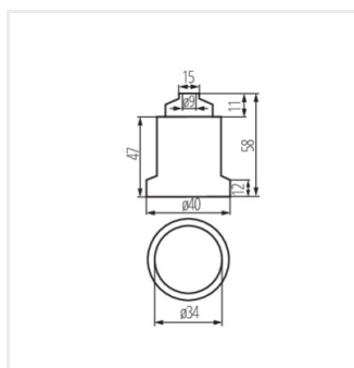
HLDR-E27-D
