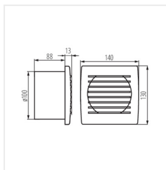
CYKLON EOL100
