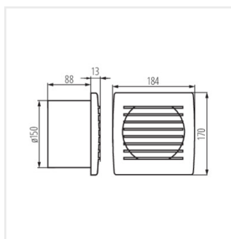
CYKLON EOL150
