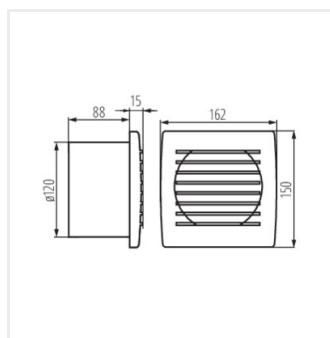
CYKLON EOL120
